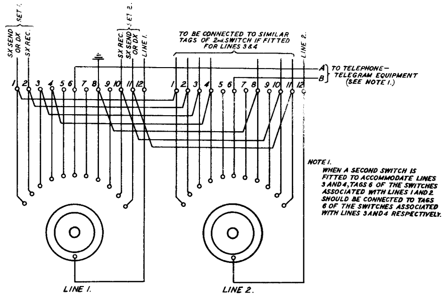
FIG. 1 WIRING
