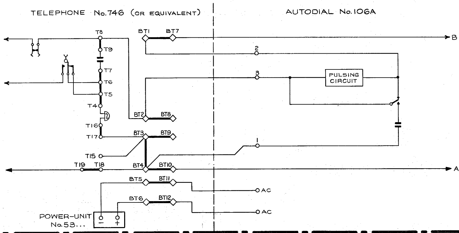
FIG.2b WIRING
