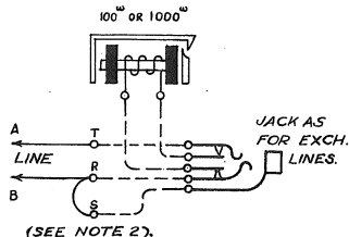
FIG. 4. CORD CIRCUIT.
