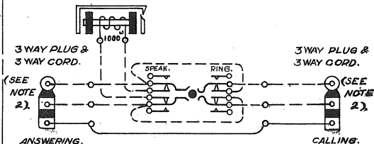
FIG. 4. CORD CIRCUIT.
