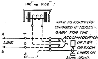
FIG. 4. CORD CIRCUIT.
