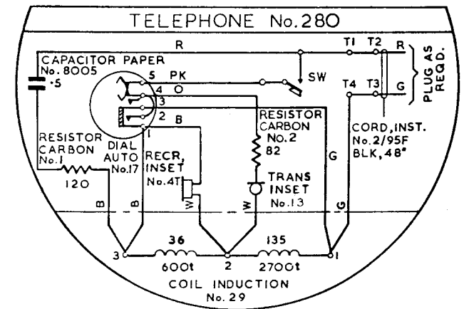
WIRING
