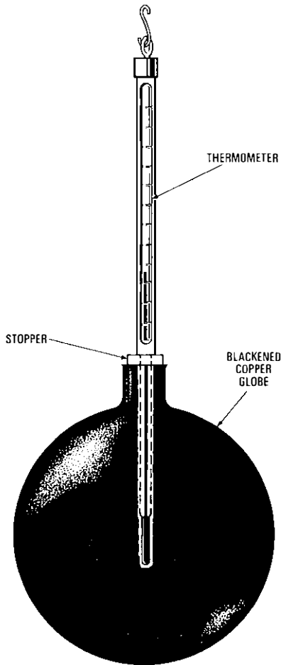
FIG. 1—Globe thermometer
