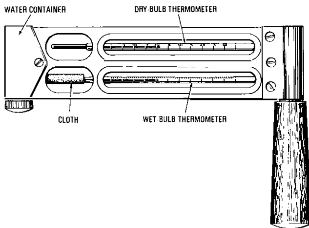
FIG. 2—Sling psychrometer
