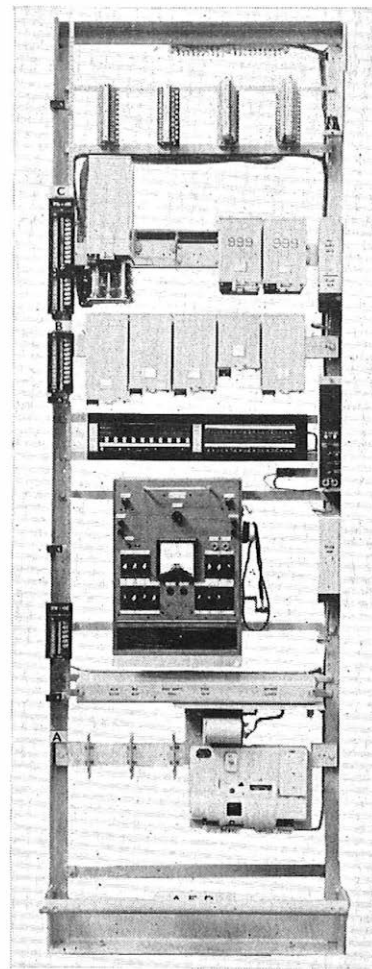
FIG. 4—ALARM-EQUIPMENT RACK
