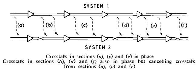
FIG. 5—PHASE-INVERSION CONNEXIONS
