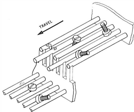
FIG. 7—SIEVING SECTION
