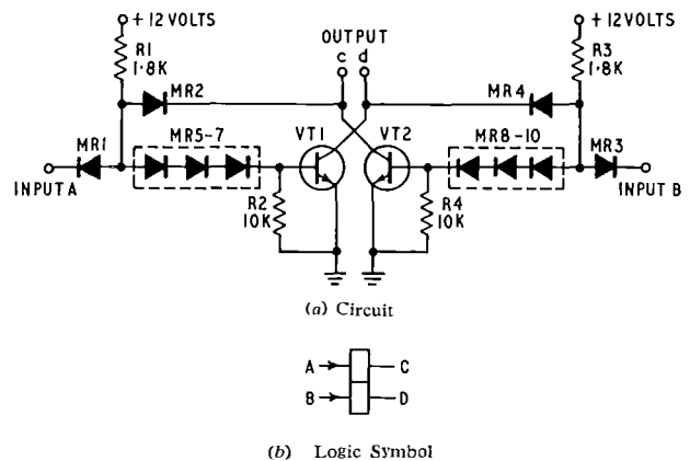
FIG. 34—TOGGLE CIRCUIT
