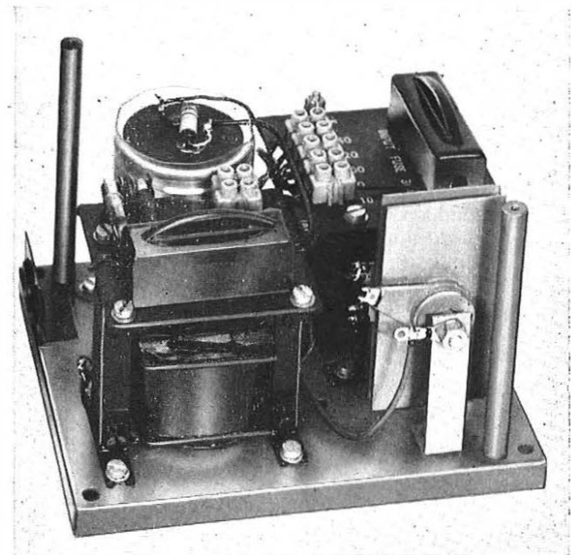
FIG. 5—POWER UNIT
