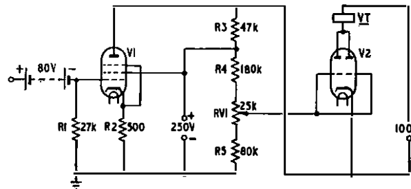
FIG. 6—VALVE-VOLTMETER CIRCUIT
