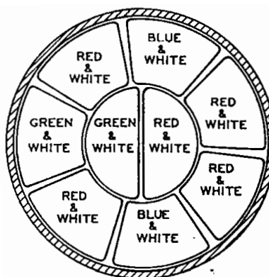
FIG. 1.—909-PAIR AMERICAN TYPE UNIT CABLE (½ LB.).
