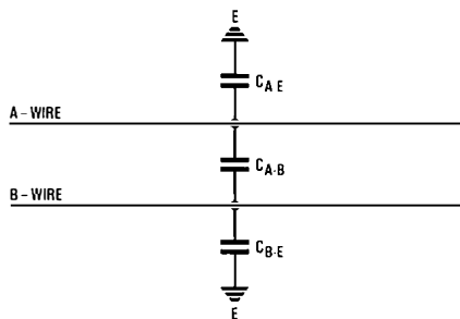
FIG. 4—Line capacitances
