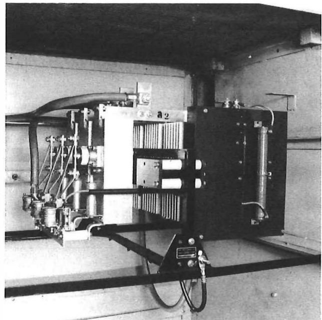
FIG. 7—New silicon rectifier unit
