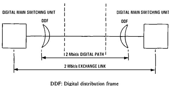
FIG. 1—Digital-digital circuit
